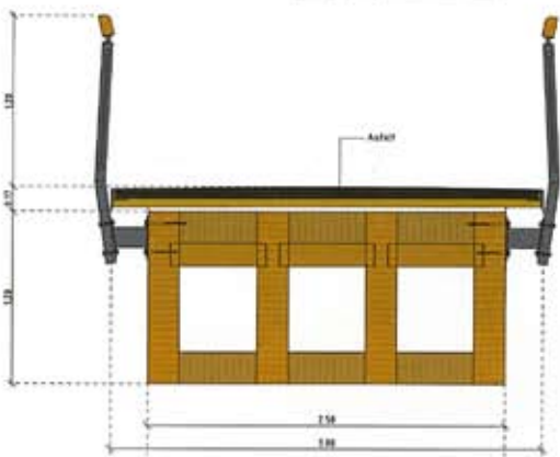
Doorsnede Meerlobrug.
