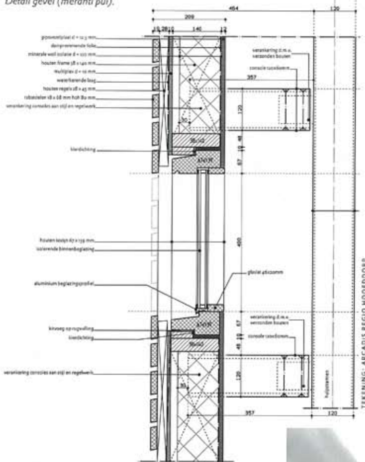
Detail gevel (meranti pui).
